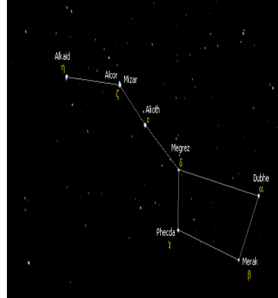
تظهر النسبية العامة بان الضوء يجب ان ينحني تحت تأثير حقول الجاذبية، والشكل اعلاه يوضح كيف ان كتلة الشمس (A) تنحني المسح الزماني - التلقائي، والتمثيل القريب منها مما يجعل الضوء المسافر من نجم بعيد (B) ينحرف حين مروره بالقرب من الشمس هذا الامر يؤدي الى ان الرقيب من الأرض (C) يتوهم ان موقع النجم هو (D) بدلا من (B).
